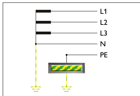
Fig. 46: TT system
