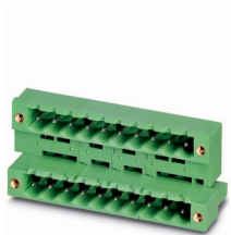
MDSTB 2,5/12-GF
