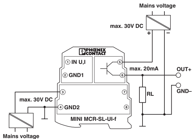
Figure 9 MINI MCR-SL-UI-F...
