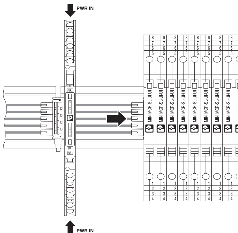
Figure 1-3 Supply via any other MACX Analog, MINI Analog or MINI Analog Pro power terminal block
