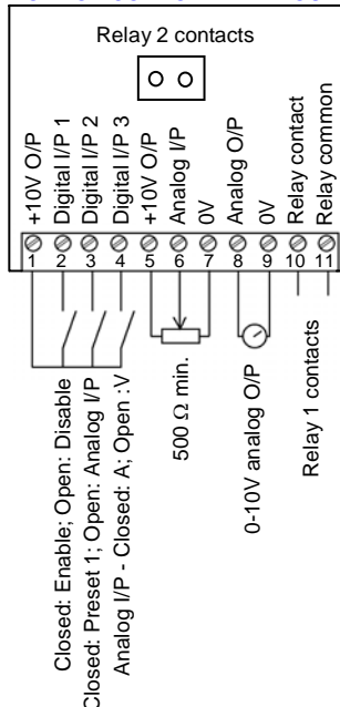
Optidrive size 2
