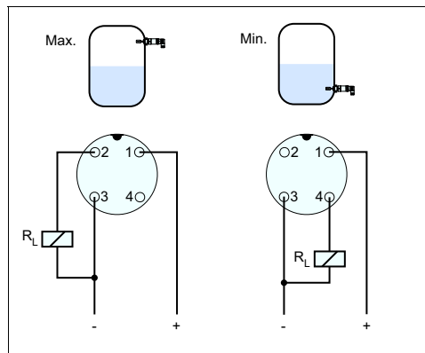
Abb. 8: Anschlussplan (Gehäuse), Transistorausgang bei M12 x 1-Steckverbindung
