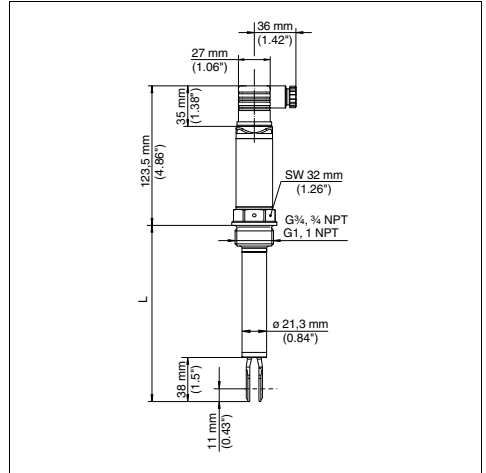
Abb. 12: LFV 230, Hochtemperaturlausführung mit Ventilstecker nach ISO 4400 L = Sensorenlänge, siehe Kapitel "Technische Daten"
