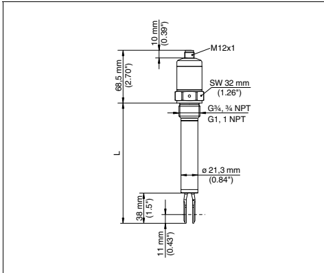
Abb. 10: LFV 230, mit M12 x 1-Steckverbindung L = Sensorenlänge, siehe Kapitel "Technische Daten"
