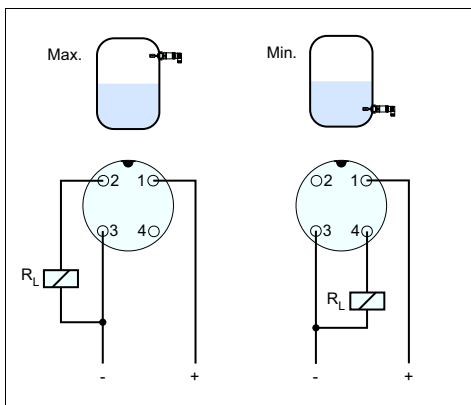
Fig. 44: Esquema de conexión (carcasa), salida de transistores de la conexión de enchufe M12 x 1
