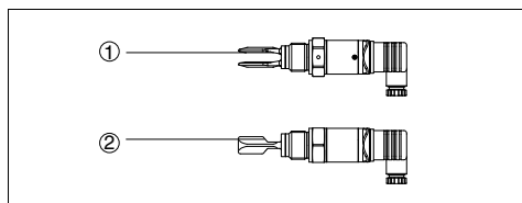
Fig. 38: Montaje horizontal
