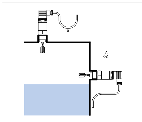
Abb. 3: Maßnahmen gegen das Eindringen von Feuchtigkeit
