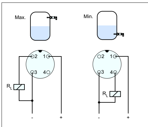
Fig. 32: Schéma de raccordement (boîtier), sortie transistor avec connecteur mâle-femelle M12 x 1
