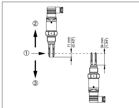
Fig. 37: Montaje perpendicular
