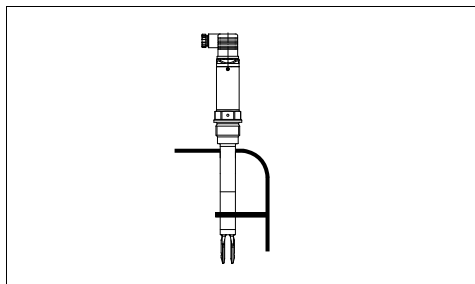
Fig. 41: Soporte lateral del LfV 230
