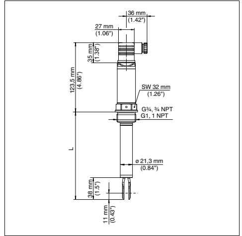
Fig. 48: LFV 230, versión de alta temperatura con enchufe de válvula DIN 4400 L = Longitud del sensor, ver capítulo "Datos técnicos"
