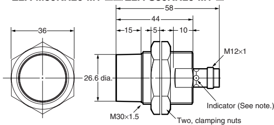
E2A-M30KN20-M1-□□/E2A-S30KN20-M1-□
