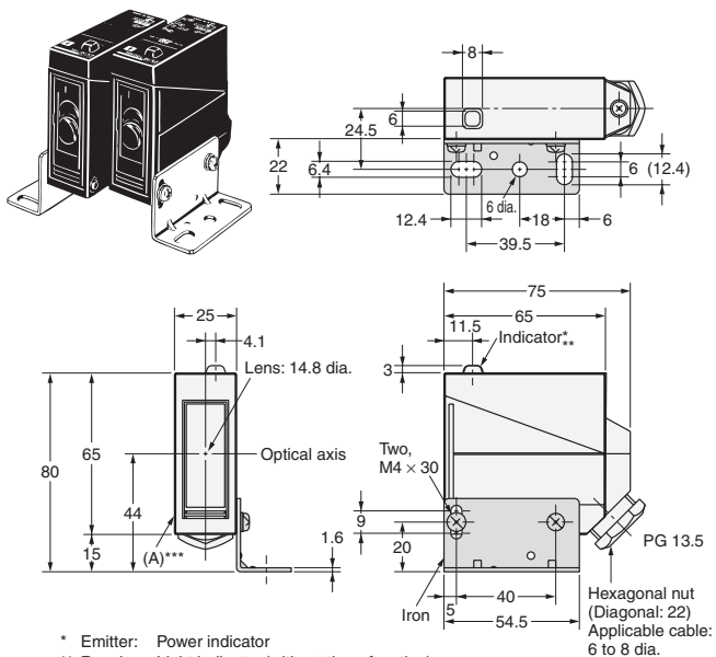
E3JM-10□4T
