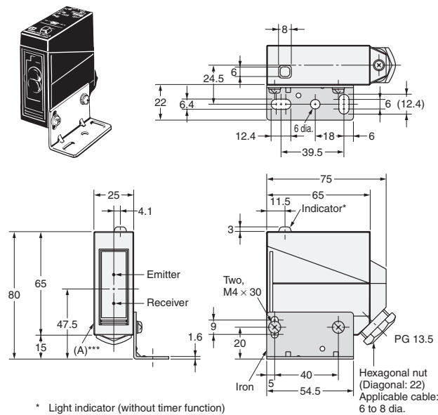
E3JM-DS70□4(T) E3JM-R4□4(T)
