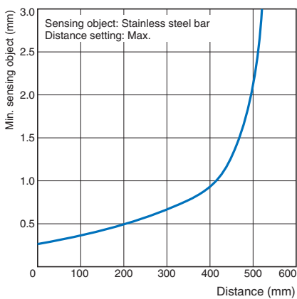
E3S-CL1 Horizontal
