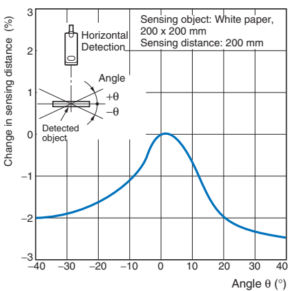
E3S-CL2 Horizontal
