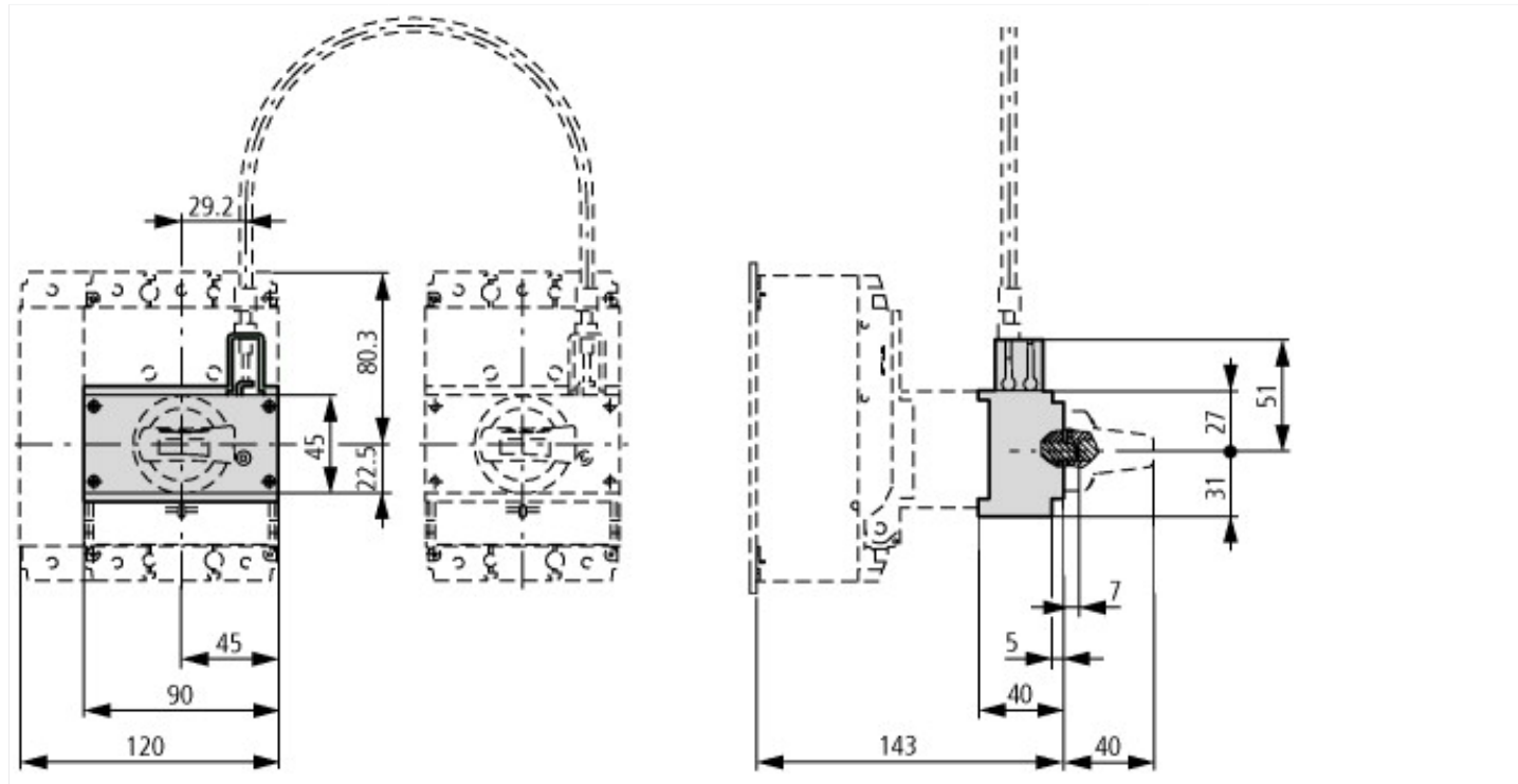
NZM1-XMV + NZM1-XDV(R)
