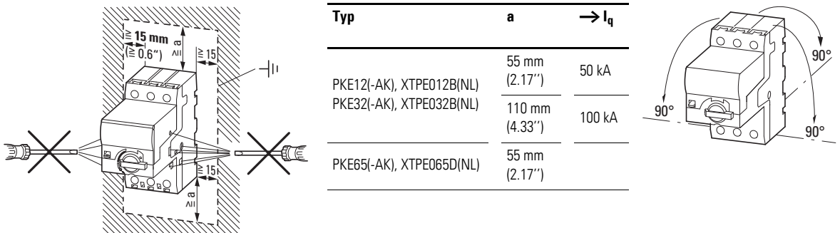
Abbildung 9: Zugelassene Einbaulage für Motorschutzschalter PKE
