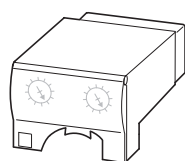
Abbildung 1: Komponenten des Motorschutzschalters PKE
