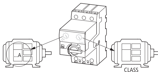
Abbildung 4: Einstellrad für Motornennstrom
