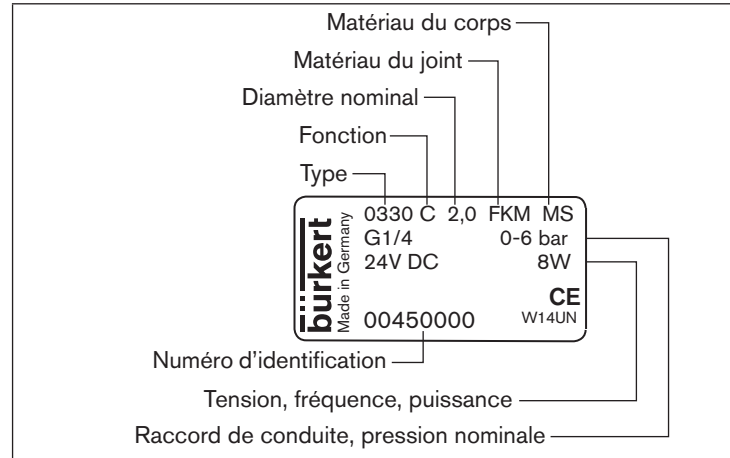
Fig. 1 : Description de la plaque signalétique
