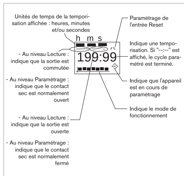
Fig. 13 : Afficheur du 1077-2
