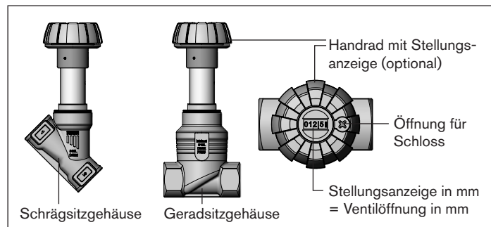
Bild 2: Ventiltypen
