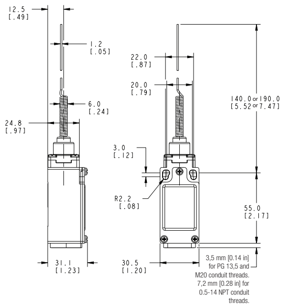
Figure 11. GLC Conduit
