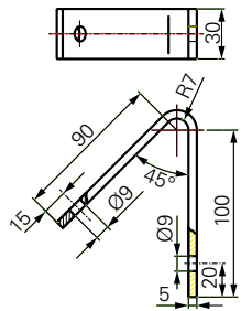
Wandbügel 45°
