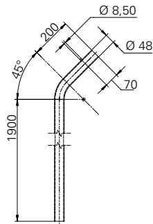
LM 48 - 1900/190 - FT
