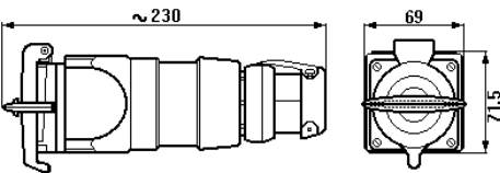
Prolongateur, GHG 513
