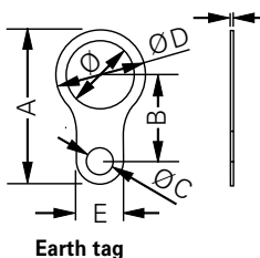
Earth tag
