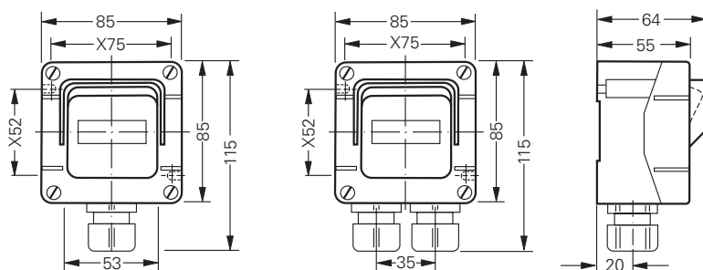
Switch/pushbutton
