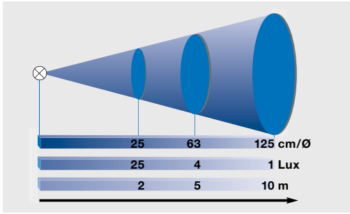
Range-diagram Stabex mini LED
