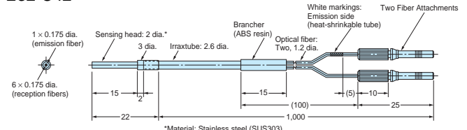
E32-C42
