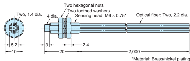
E32-D22L
