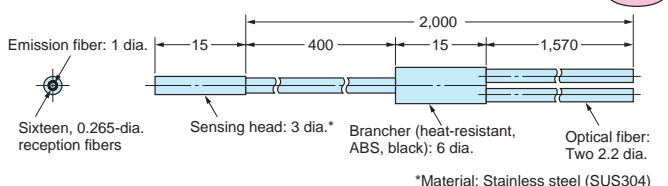
E32-D32L
