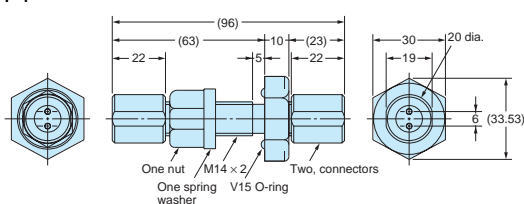
E32-VF1
