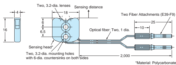
E32-L25A
