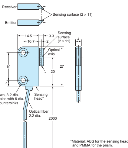
E32-T16J E32-T16JR
