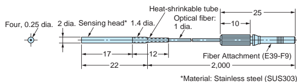
E32-T22B
