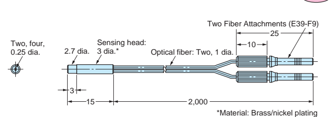
E32-D15XB
