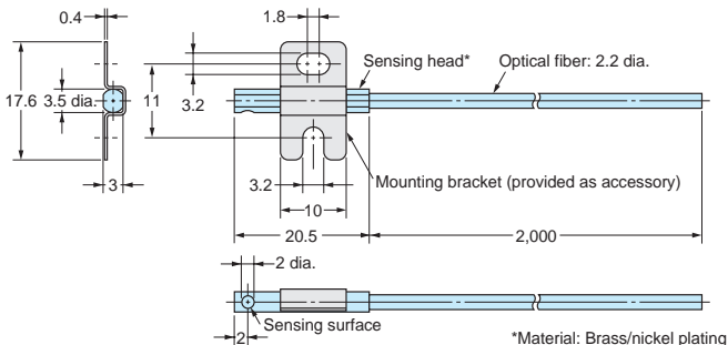
E32-M21
