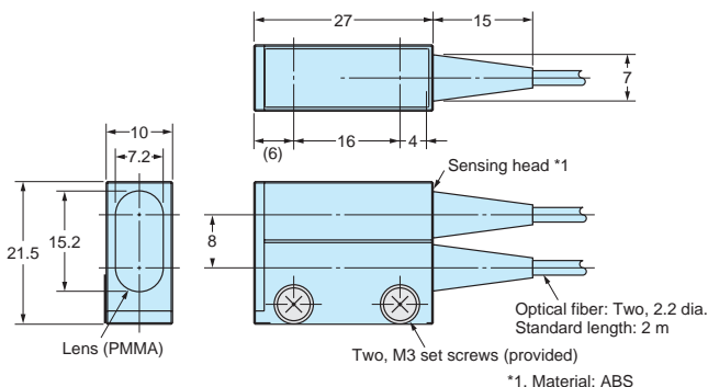
E32-R16
