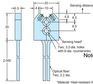
E32-L25A
