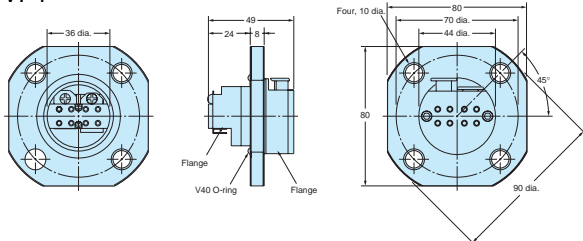
E32-VF4
