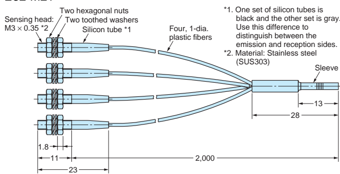
E32-T16
