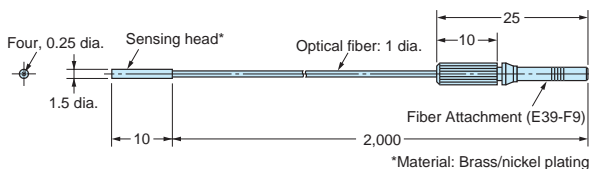
E32-T25XB
