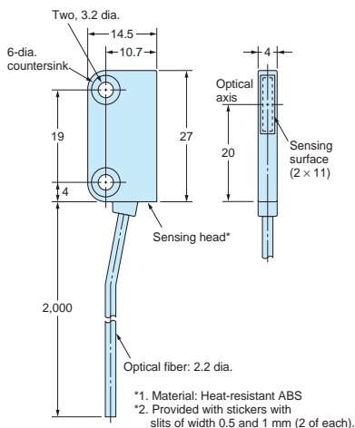
E32-T51
