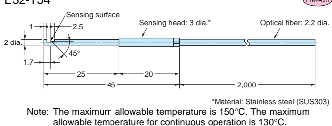
E32-T54
