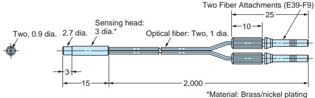
E32-D22L
