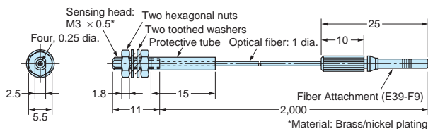
E32-T221B
