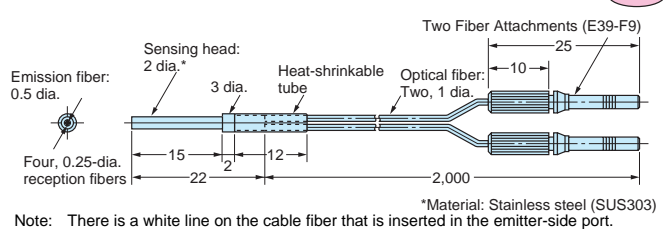
E32-C42
