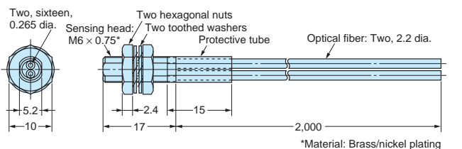
E32-D21B
