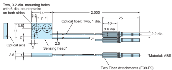
E32-L24L
