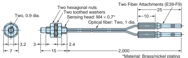
E32-D21L
