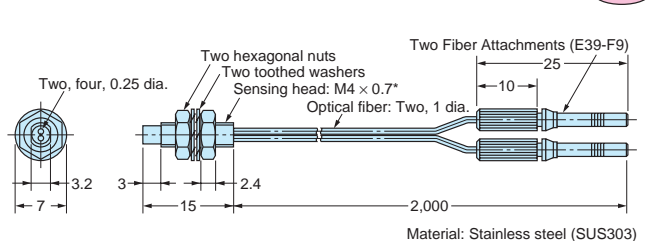
E32-D221B
