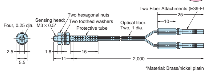
E32-D22B
