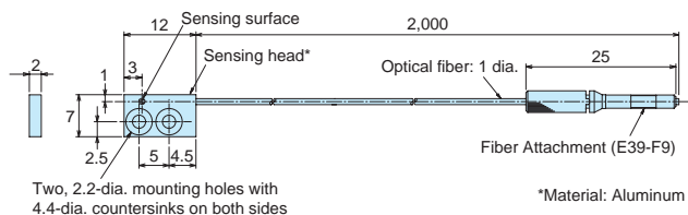
E32-T25Z E32-T25ZR
