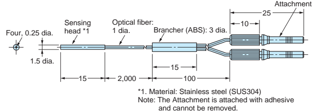
E32-D25XB
