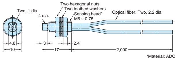
E32-DC200 E32-D11R
