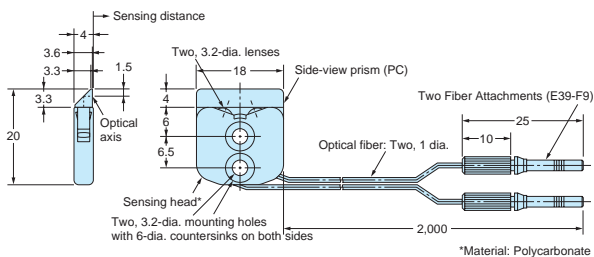
E32-L25
