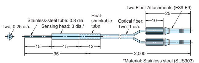
E32-D33
