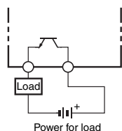
PNP Output
