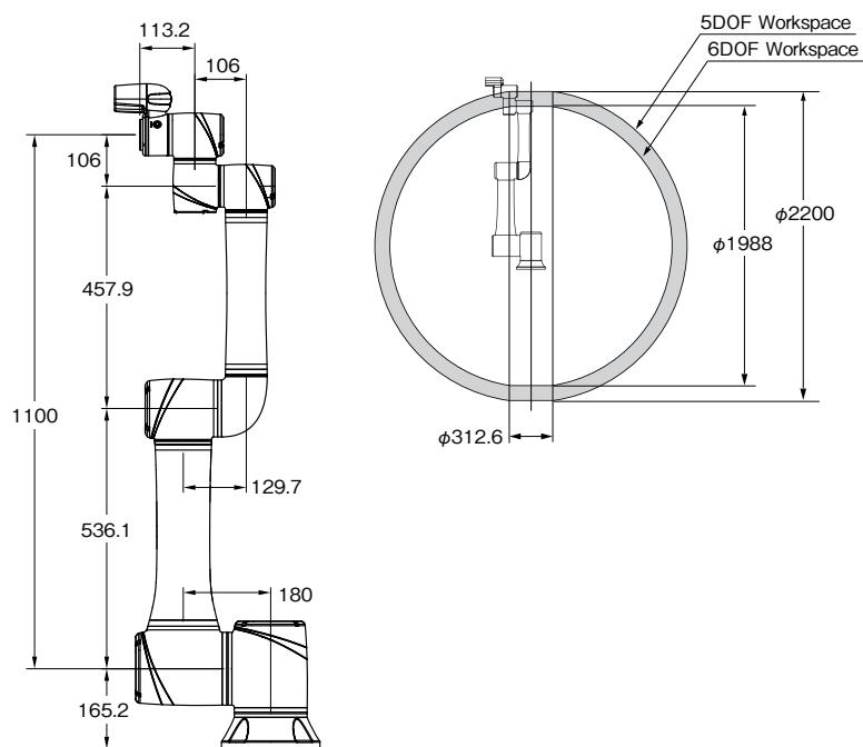
TM14
