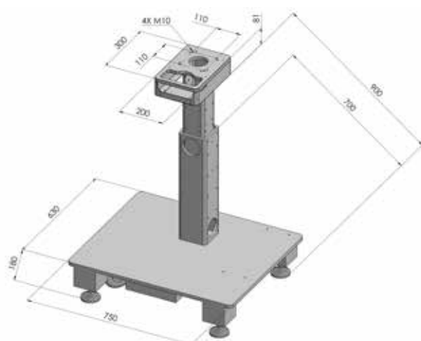
Robot Stand
