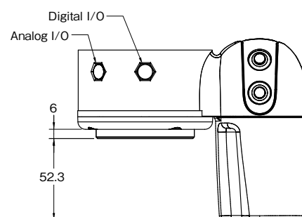
Flange
