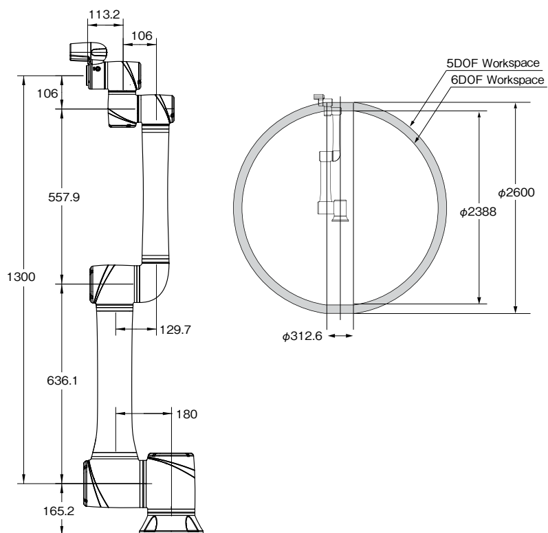
TM12
