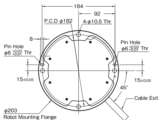
Flange
