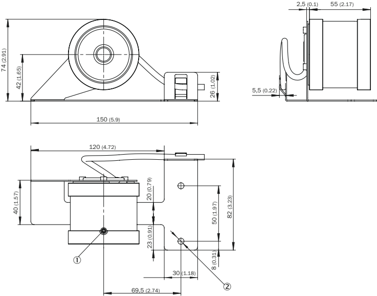
Abbildung 5: DKV60 mit Rndel Messradoberflche
