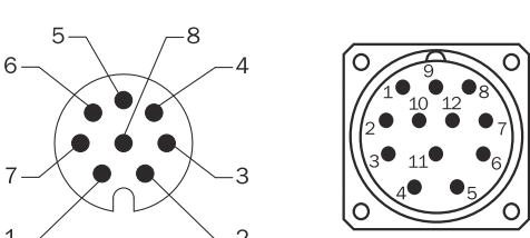
Abbildung 7: Ansicht Gertestecker M12 / M23 an Leitung / Gehuse
