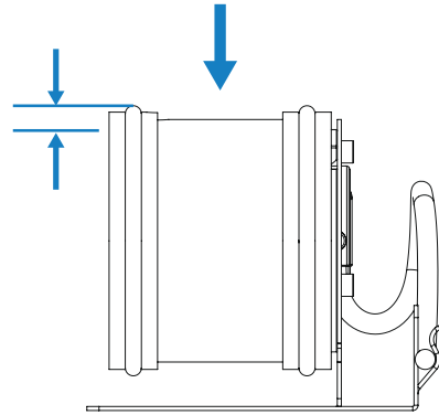
Abbildung 2: Betriebsposition / Federkraft = 2 ... 5 mm (5 ... 10 N)
