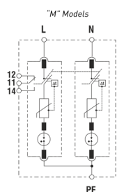
TNS LF (1Ph+N) - 2P
