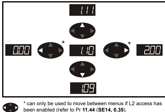
Figure 1-1 Parameter navigation
